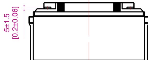
B5 Terminal
