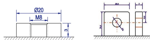
M8 Bolt
